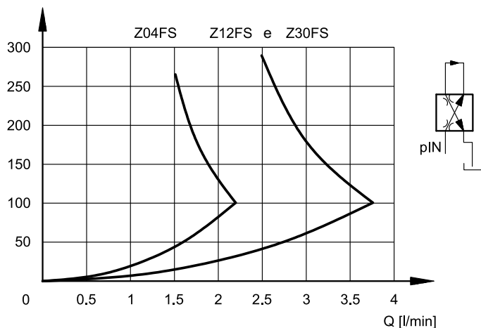
CURSORE Z*FS - FUNZIONE FAIL SAFE
